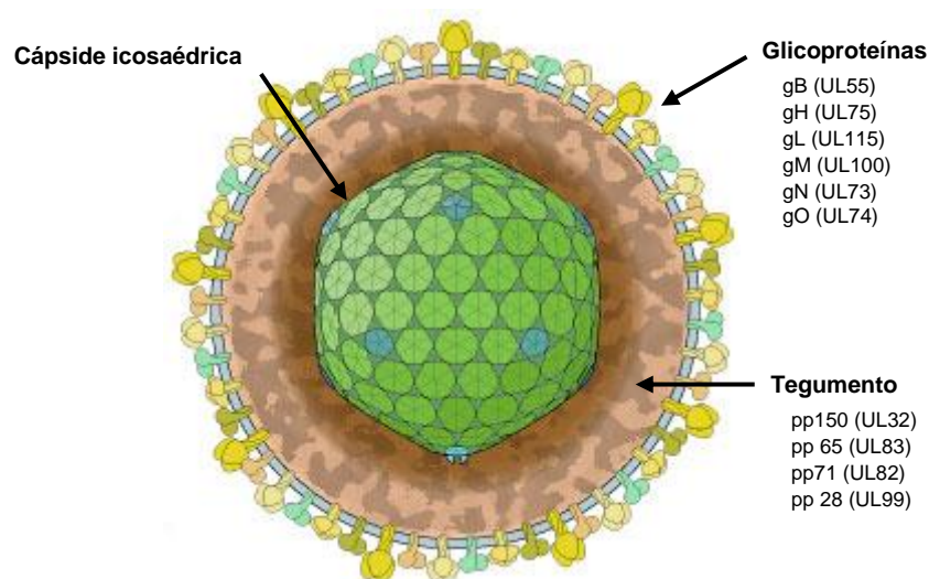
Figura 5 - Estrutura do CMV com as principais proteínas estruturais (Adaptado de Hulo et al, 2011)
