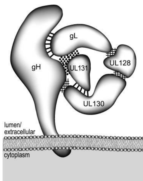
Figura 6 - Complexo pentamérico das proteínas UL128, UL130, UL131, gH e gL do CMV (Ryckman et al, 2008)
