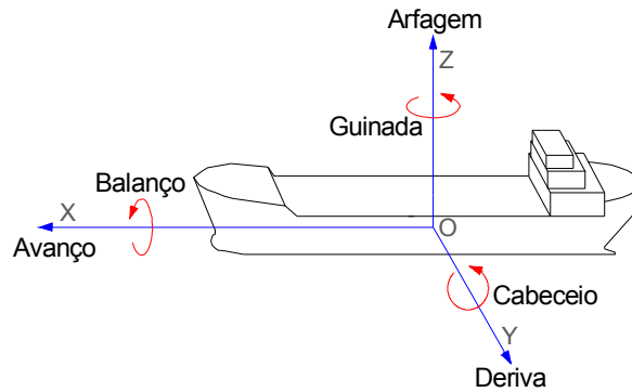
Figura 11 – Movimentos de um navio amarrado.
