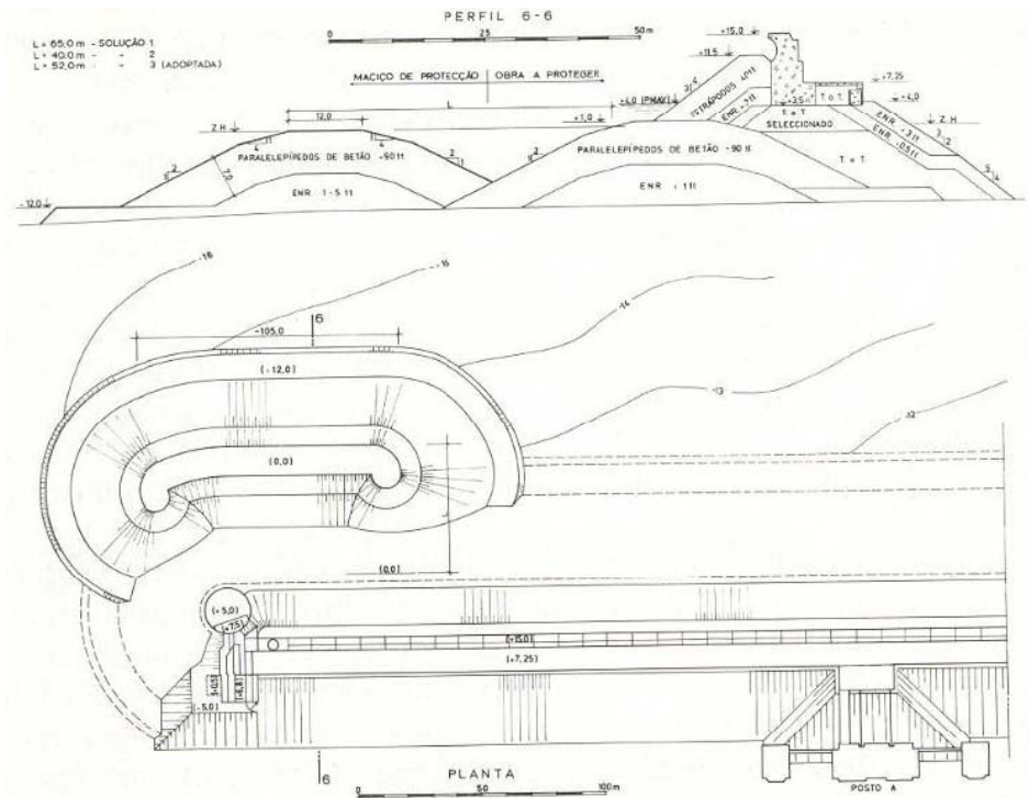
Figura 7 – Cabeça do quebramar Norte do Porto de Leixões (Vera-Cruz e Carvalho, 1993).
