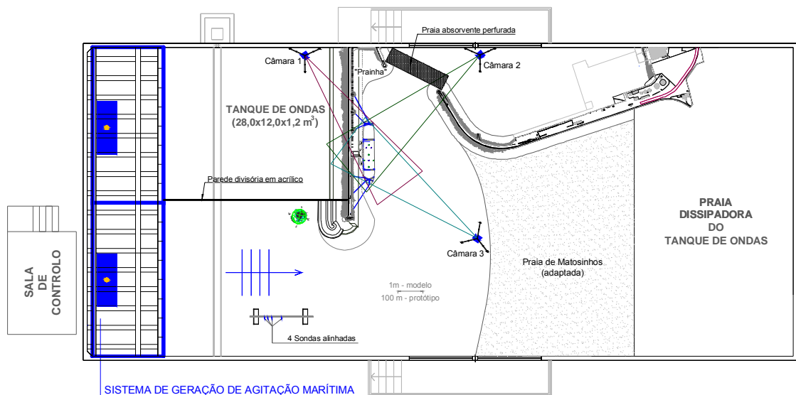
Figura 9 – Esquema de implantação do modelo físico no tanque de ondas: 2 a fase do estudo.
