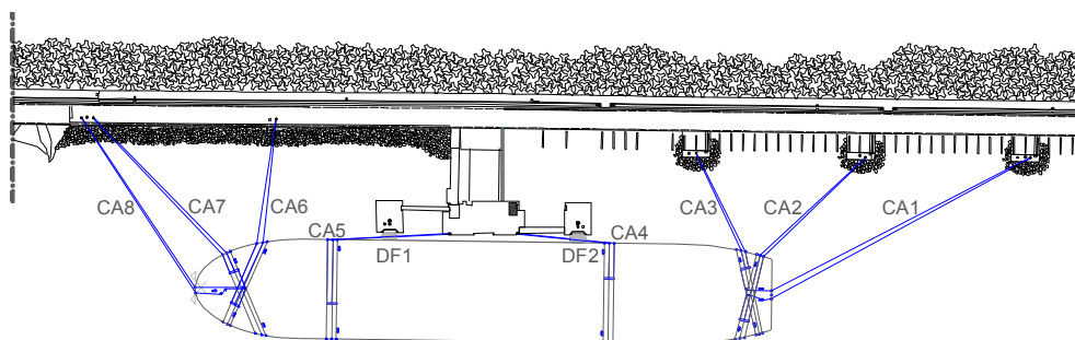
Figura 3 – Layout de amarração do navio, com identificação dos cabos de amarração e defensas.
