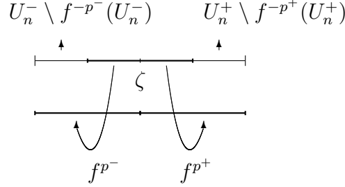
Fig.7 - Q_{p^-, p^+}(u_n) = \left( U_n^- \setminus f^{-p^-}(U_n^-) \right) \cup \left( U_n^+ \setminus f^{-p^+}(U_n^+) \right)
