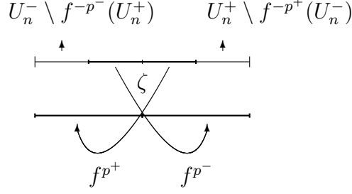
Fig.9 - Q_{p^-, p^+}(u_n) = \left( U_n^- \setminus f^{-p^-}(U_n^+) \right) \cup \left( U_n^+ \setminus f^{-p^+}(U_n^-) \right)
