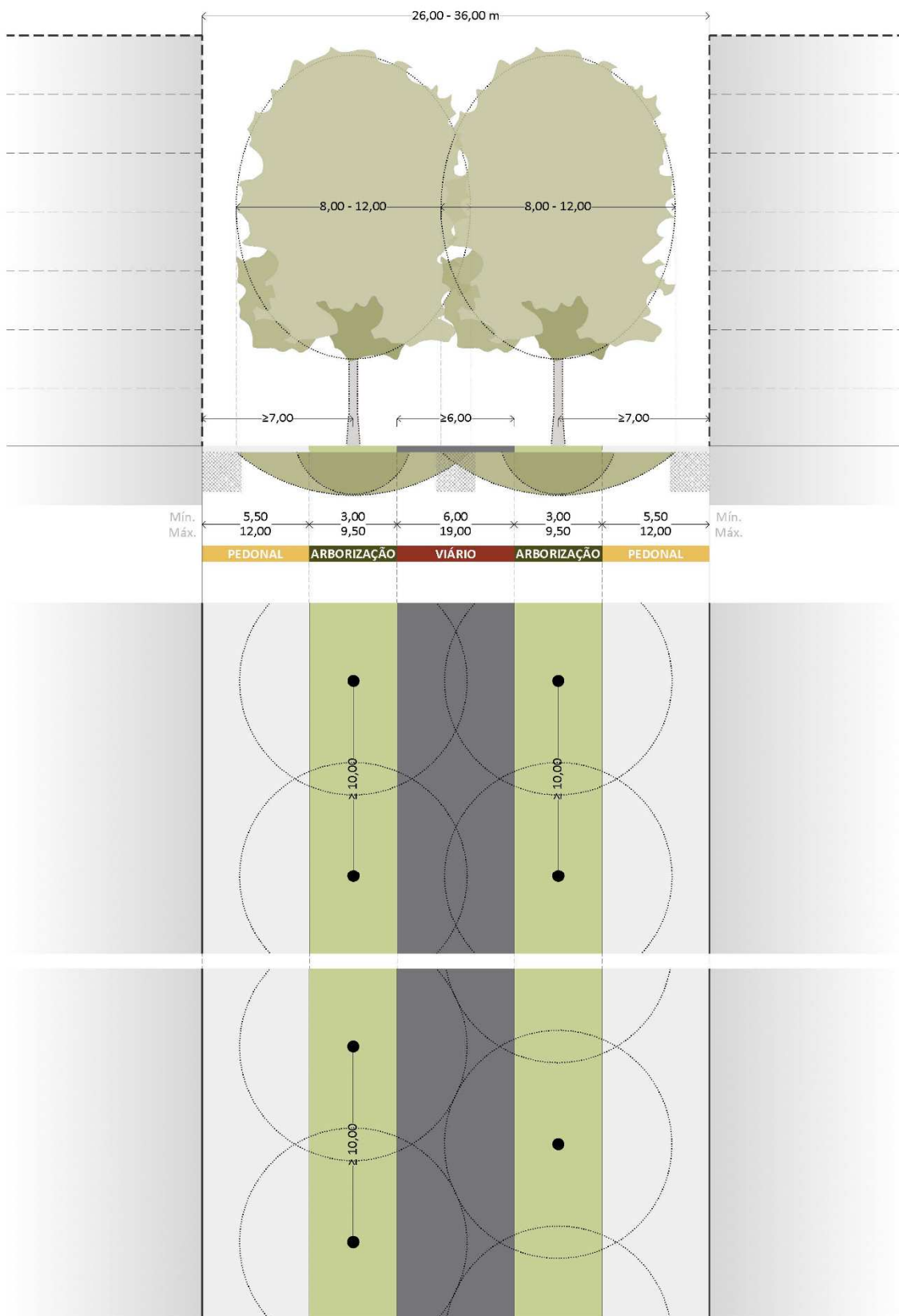
Figura 5.30 – Representação do modelo 10, em corte e em planta.
