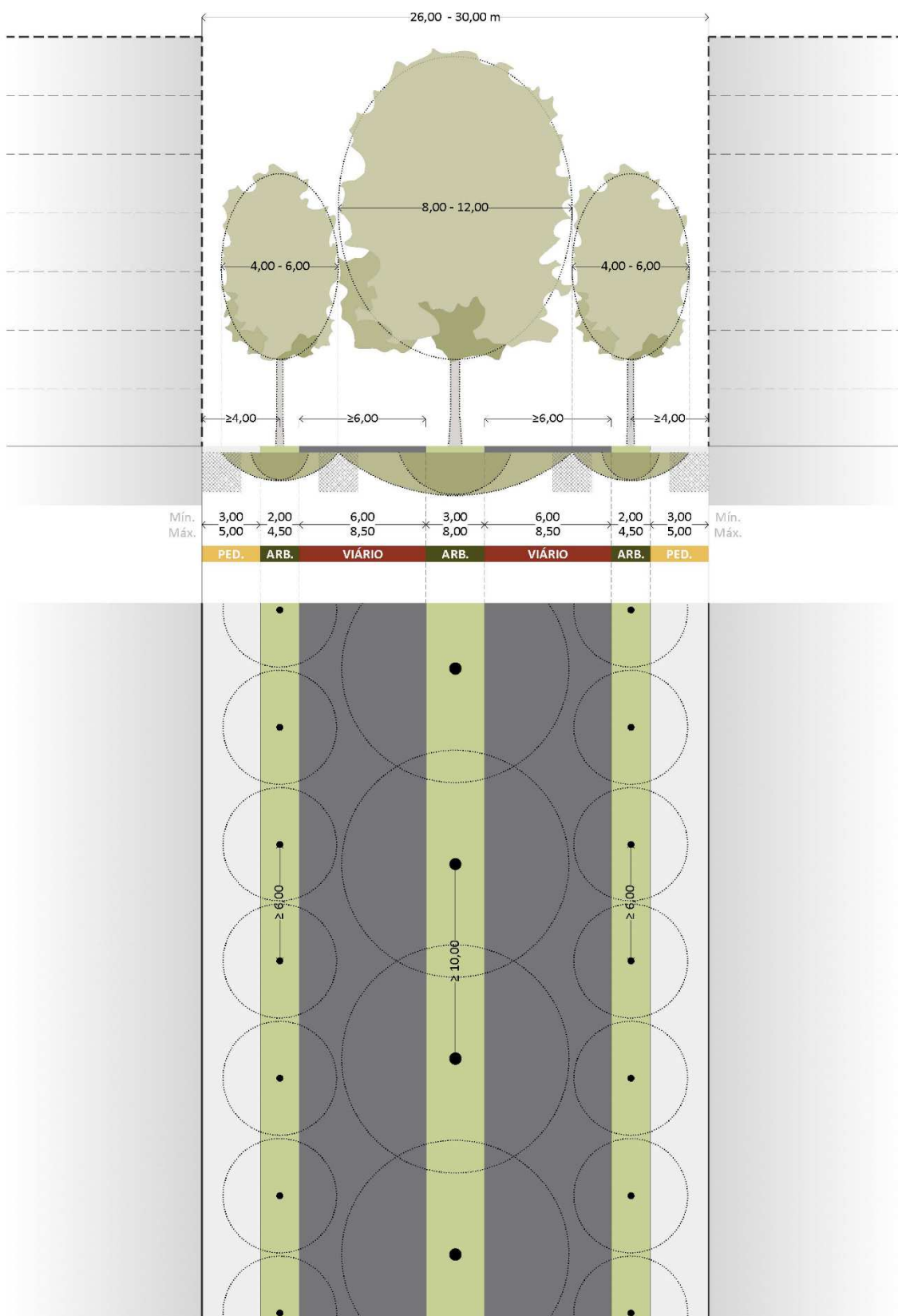
Figura 5.32 – Representação do modelo 12, em corte e em planta.
