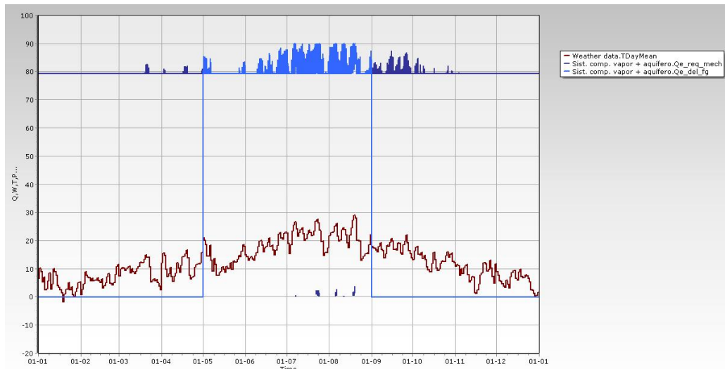
Fig.8 | Potências frigoríficas (kW) retiradas do espaço ao longo do ano com o sistema de compressão de vapor acoplado ao aquífero.
