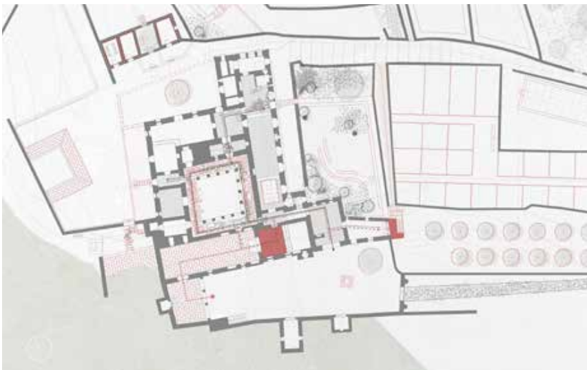
Planta do piso 0 (cota 131.26) | existente e proposta (vermelho). Floor plan (elevation 131.26) | existing and proposed.
