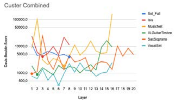
(d) Combined Clustering
