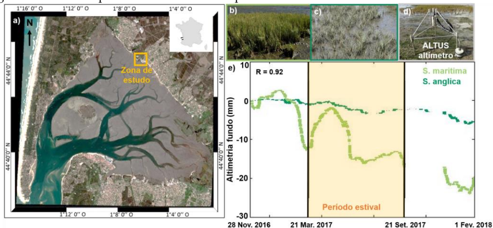
Figura 1. a) Zona de estudo; b) Spartina maritima ; c) Spartina anglica ; d) Estrutura ALTUS - altímetro acústico; e) Variação temporal da altimetria de fundo sob a influência das espécies Spartina anglica e Spartina maritima .
