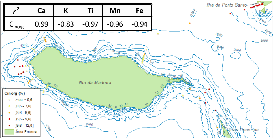
Figura 1. Distribuição espacial do teor em carbono inorgânico ( C_{inorg} ) e coeficientes de correlação de Pearson ( n=62 ) entre elementos.
