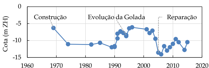
Figura 1. Profundidade máxima de erosão na vizinhança do esporão EV2 entre 1969 e 2015.
