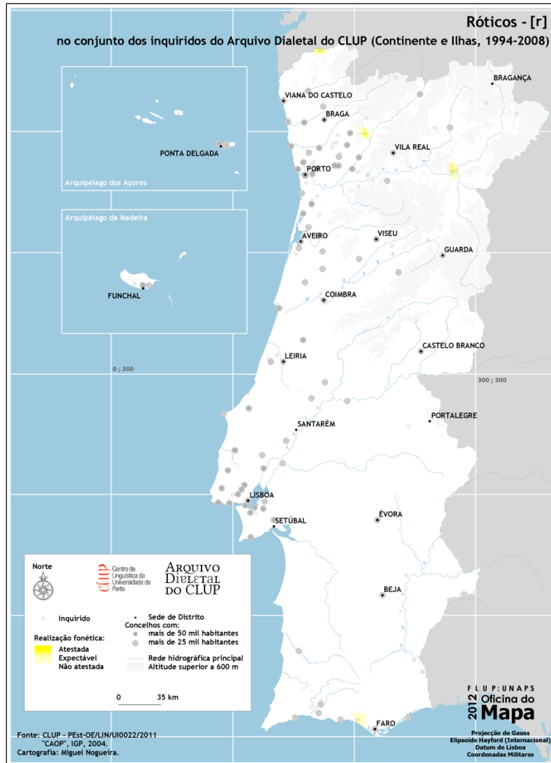
Figura 4: Distribuição geográfica da vibrante alveolar.
