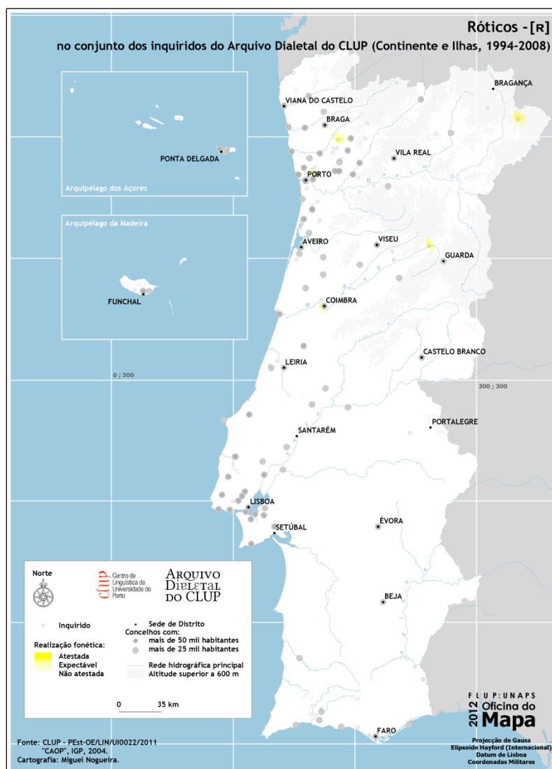
Figura 5: Distribuição geográfica da vibrante uvular.
