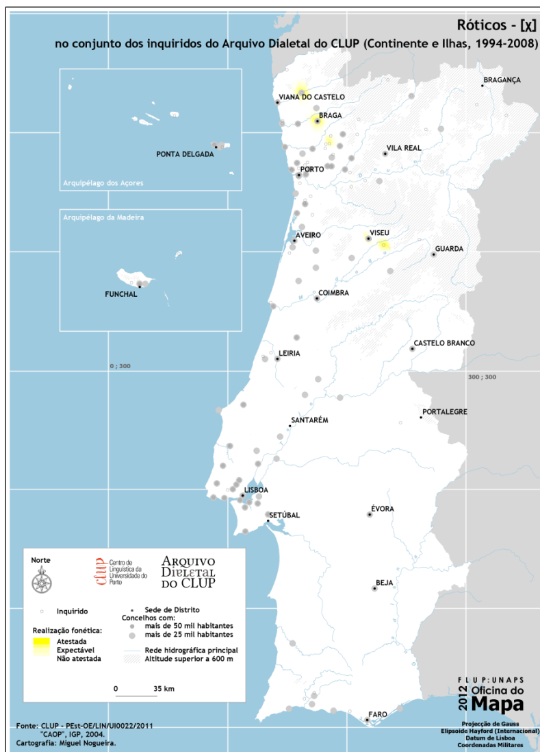
Figura 2: Distribuição geográfica da fricativa uvular surda.
