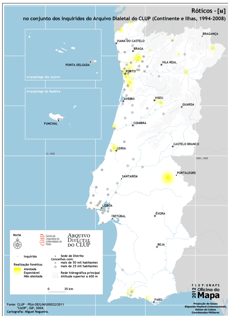
Figura 1: Distribuição geográfica da fricativa uvular sonora.
