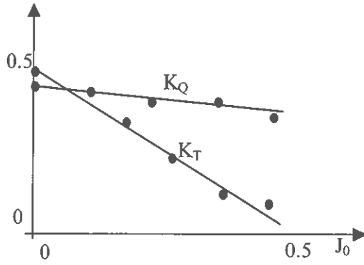
Fig. 6. Propeller parameters
