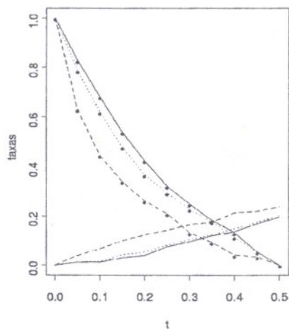
Figura 3: Taxas de erro e rejeição. Dados PIMA. Amostra de teste.
