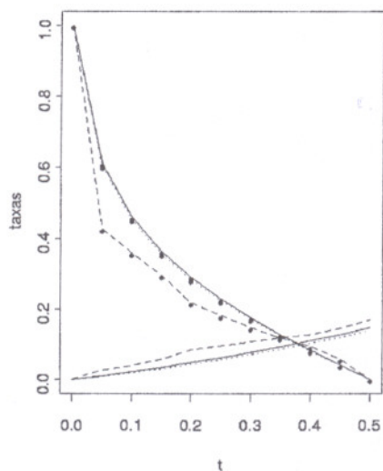
Figura 2: Taxas de erro e rejeição. Dados CHORON. LDA e Logística - "teóricas". QDA - amostra "simulada".
