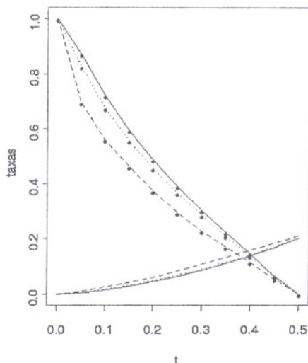
Figura 4: Taxas de erro e rejeição. Dados PIMA. LDA e Logística - “teóricas”. QDA - amostra “simulada”.
