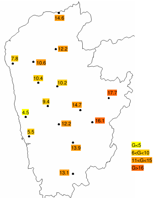
Índice de Continentalidade de Gorczyński (G)
