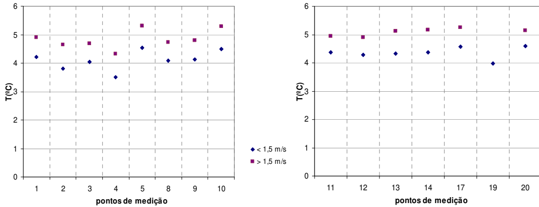
Valores médios mensais das temperaturas mínimas diárias sob abrigo, entre Fevereiro e Maio de 2004, consoante a velocidade do vento (estação de Queimadelos).
