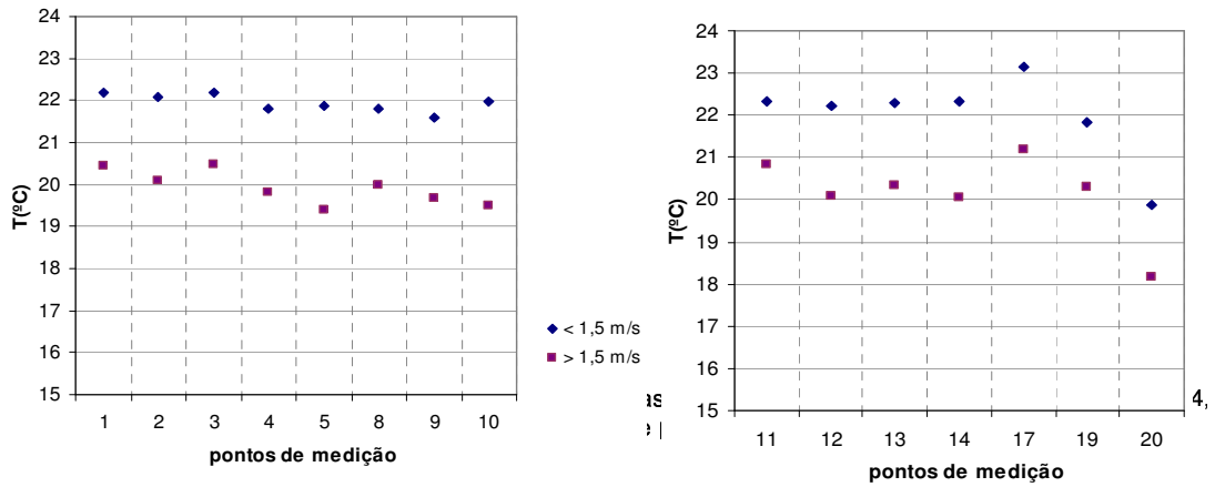
Valores médios mensais das temperaturas máximas diárias sob abrigo, entre Fevereiro e Maio de 2004, consoante a velocidade do vento (estação de Queimadelos).
