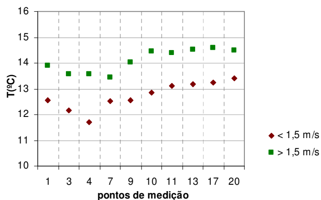
Valor médio das temperaturas máximas e mínimas diárias consoante a velocidade do vento entre Junho e Setembro (registo de Queimadelos).
